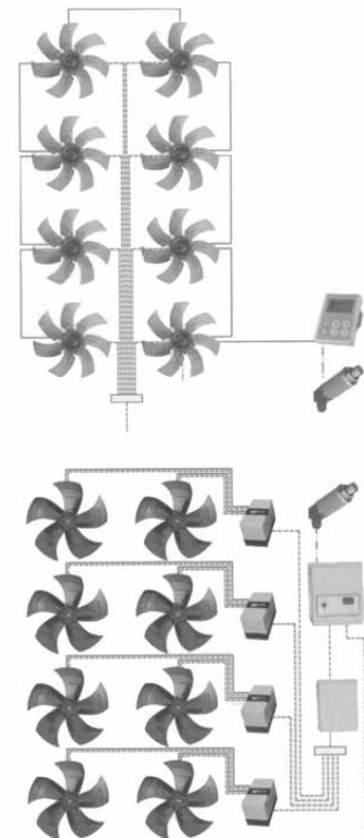
Fig 5. Configuration EC comparée à la configuration AC
